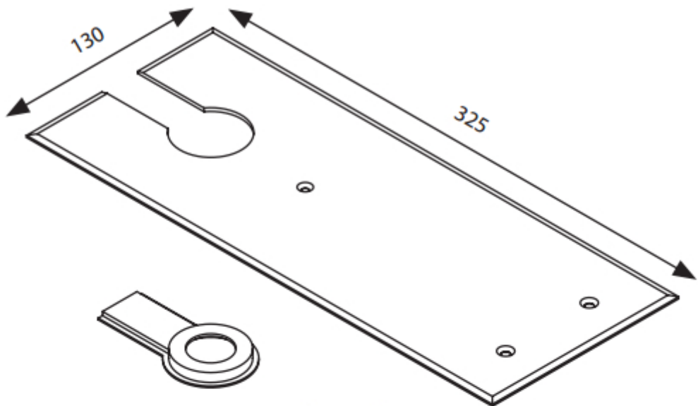
Dust Cap
